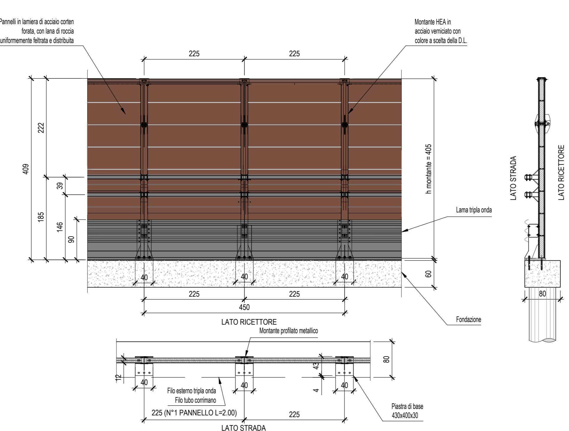
BARRIERA INTEGRATA H=4.00 m VISTA FRONTALE SCALA 1:50
