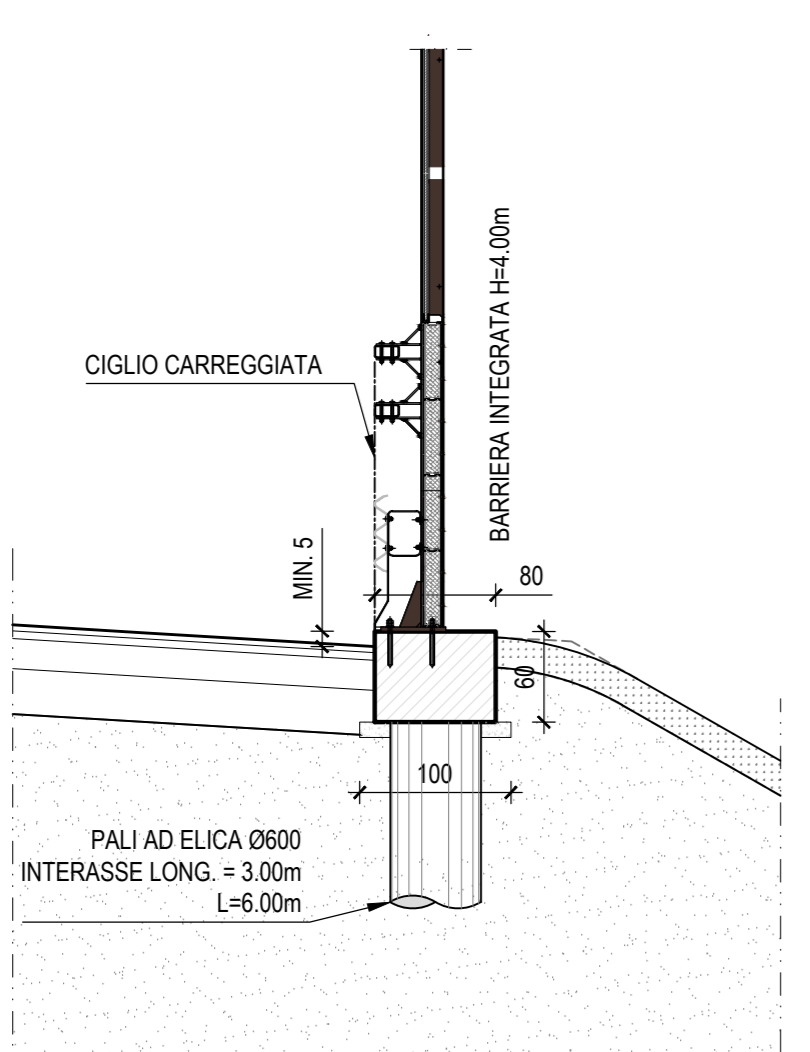
SEZIONE TIPICA SU CORDOLO BARRIERA INTEGRATA H = 4.00 m (F.O.A. 19) SCALA 1:50
