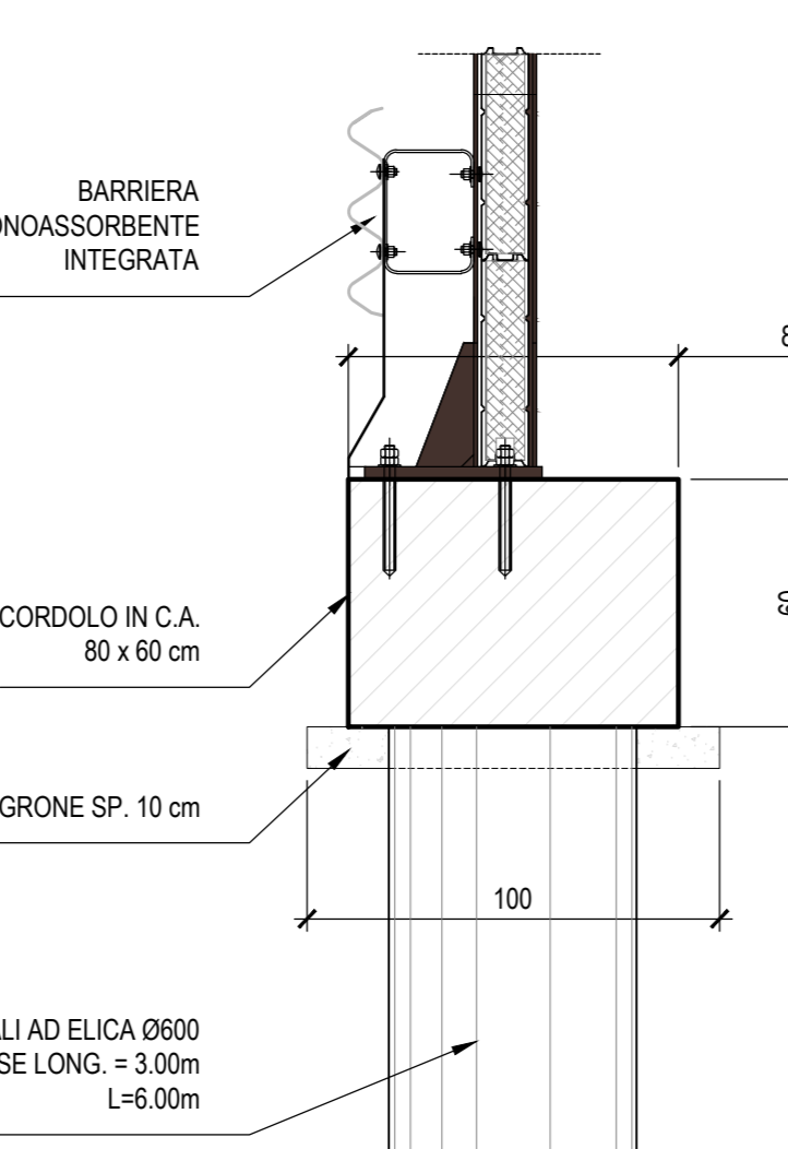
SEZIONE TIPICA SU CORDOLO CARPENTERIA SCALA 1:20
