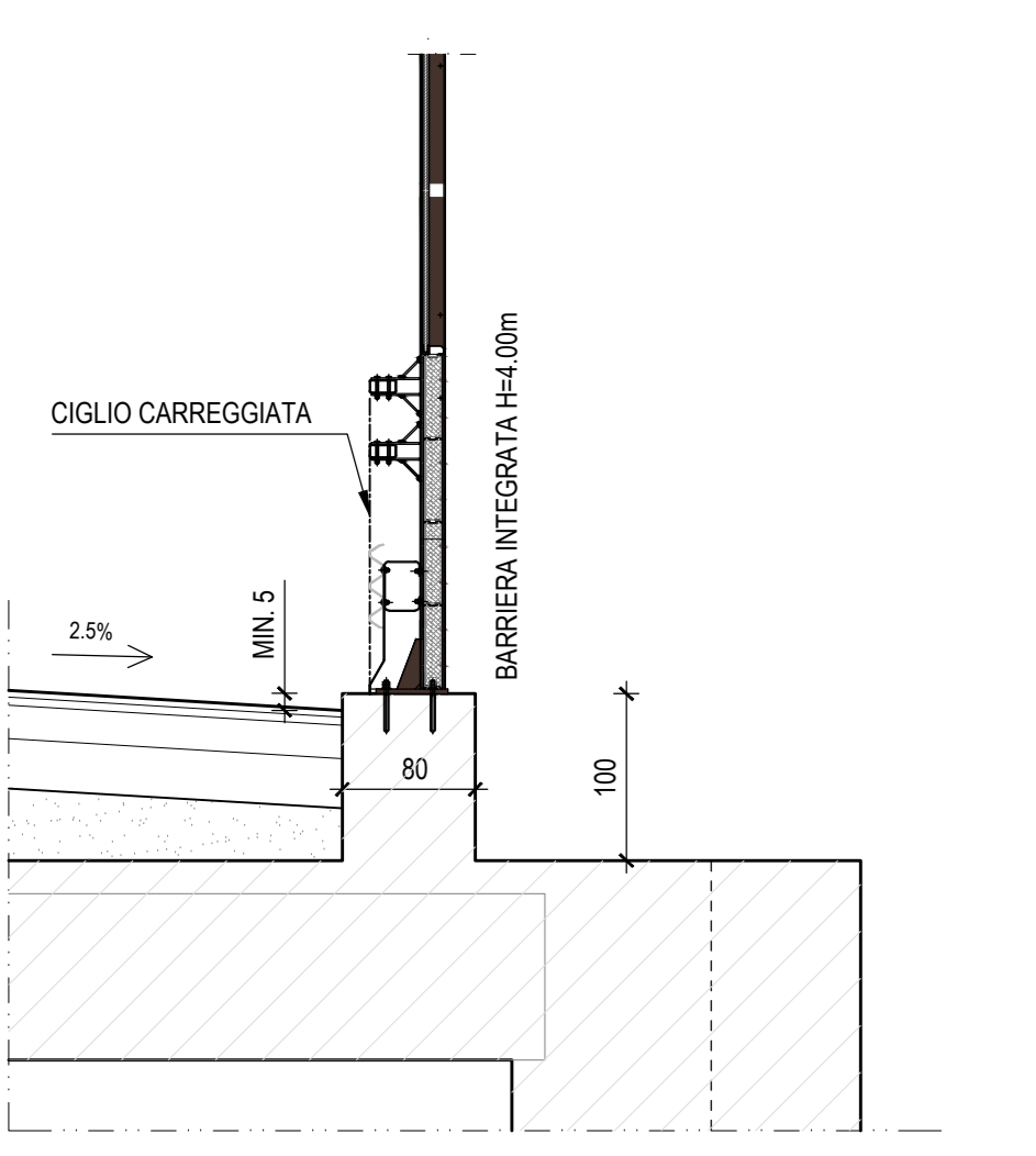
SEZIONE TIPICA SU GALLERIA ARTIFICIALE BARRIERA INTEGRATA H = 4.00 m (F.O.A. 19) SCALA 1:50
